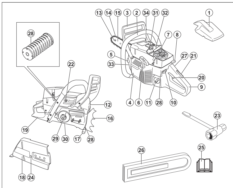
1. Luchtfilterdeksel
