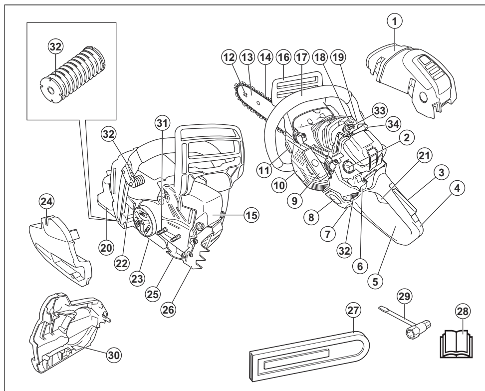
1. Cylinderkåpa
