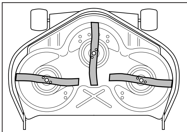
Groupe de coupe pour Rider 970 (groupe Bioclip)
