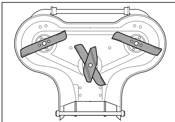
Groupe de coupe pour Rider 850 (éjecteur arrière)
