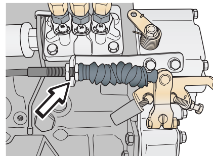
Varvtalsvajer
