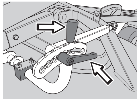
Bakre klipphöjdsinställning
