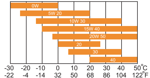
Viskositetsdiagram
