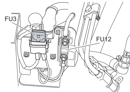
Säkringar FU3, FU12
