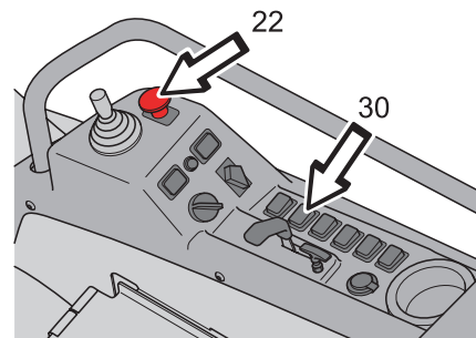
Strömställare för kraftuttag och viktöverföring
