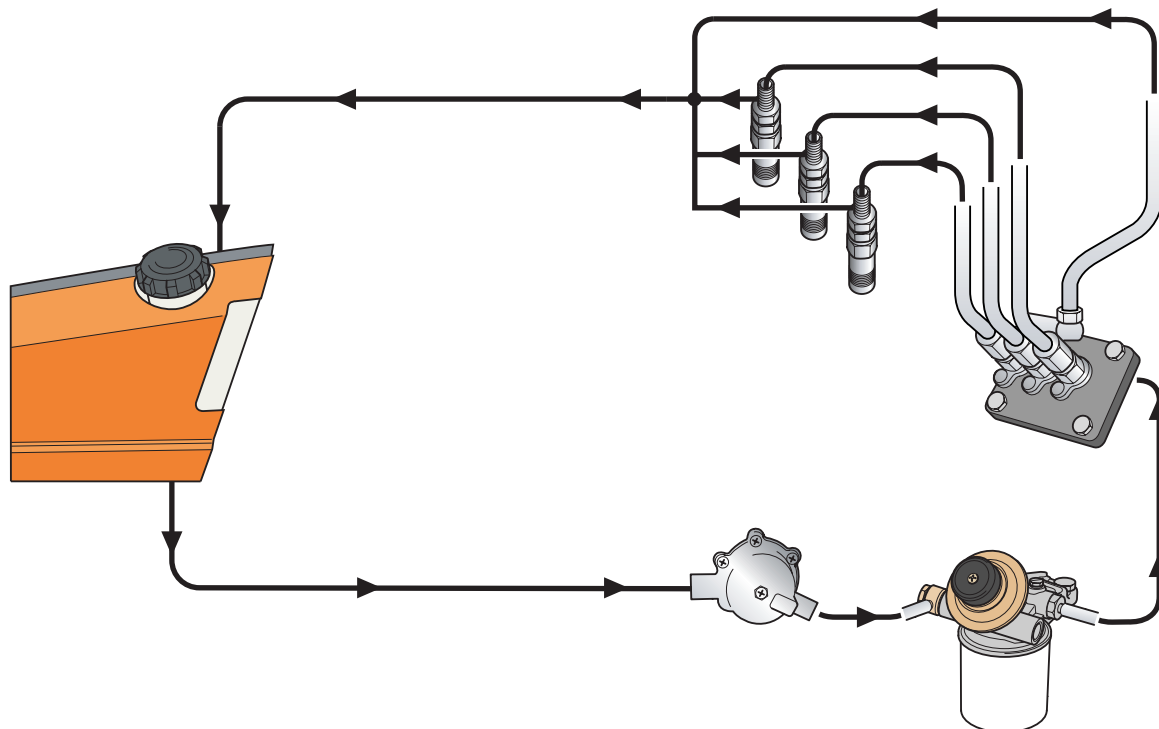
Bränslesystem
