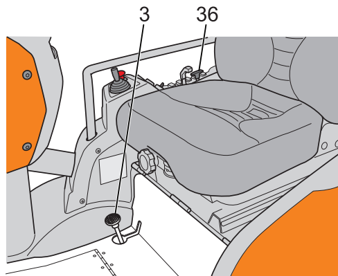
Parkeringsbroms
