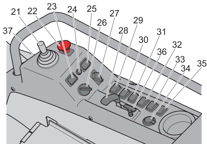
Manöverpanel
