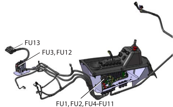
Säkringar
