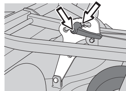
Vred klipphöjdsinställning
