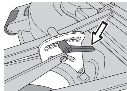
Vänster klipphöjdinställning,
