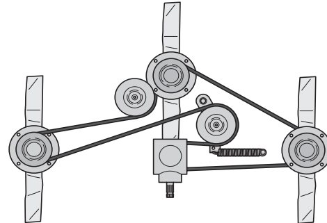
Remdragning
