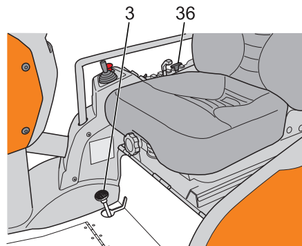
Parkeringsbroms
