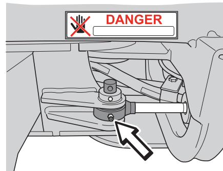
Styrcylinder
