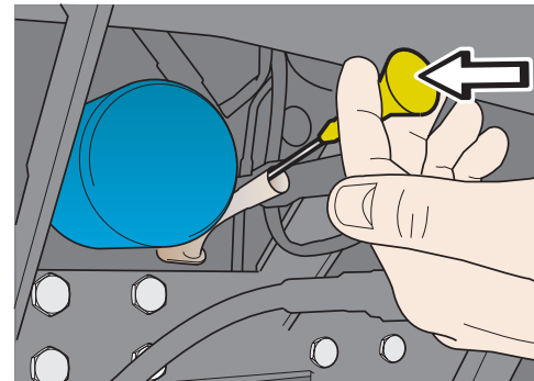
Motorns oljesticka
