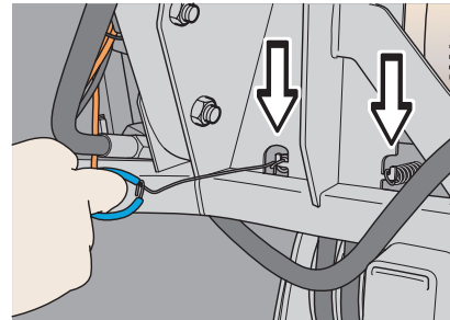
Remsträckarens fjäderfästen
