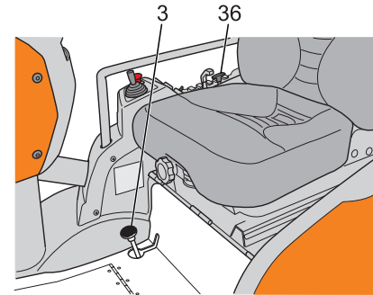
Ansätt parkeringsbroms
