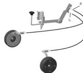
Parkeringsbromsvajrar
