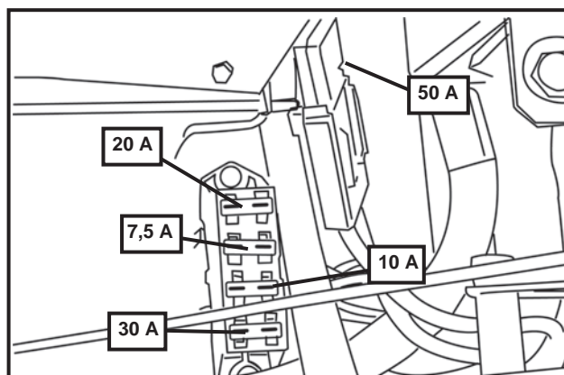
Säkringar
