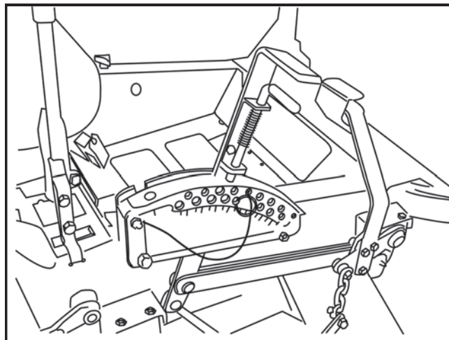
Klippaggregatets lyftspak och fotpedal
