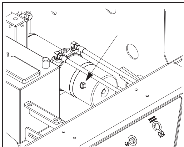
Ventilationsplugg på klippaggregatlyftens hydraulenhet
