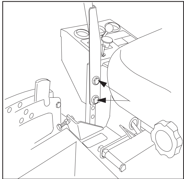
Justerskruvar
