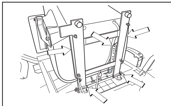
Smörj den längsgående inställningsmekanismen under stolen
