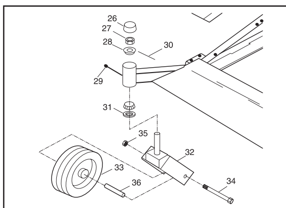
Länkhjul
