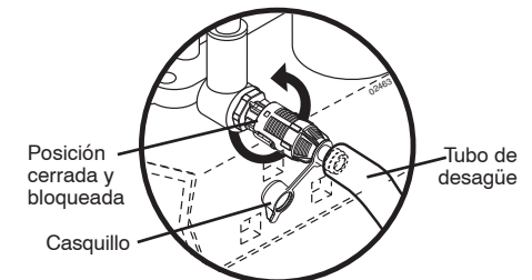
Válvula de desagüe del aceite
