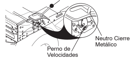
Palanca de Velocidades del Cambio Mecánico
