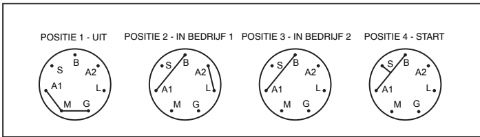
POSITIES SLEUTELSCHAKELAAR
