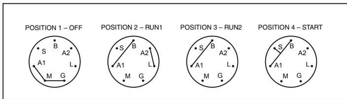
POSITIONS DE L'INTERRUPTEUR À CLÉ
