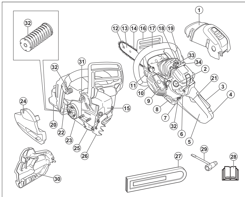
1. Sylinderdeksel
