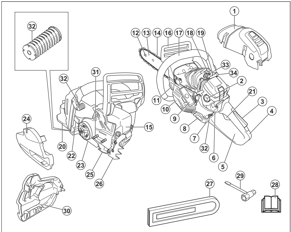
1. Cilinderkap
