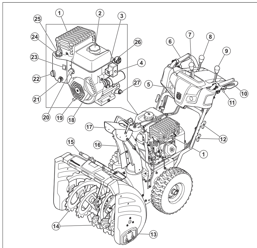
1. Lyddæmper
