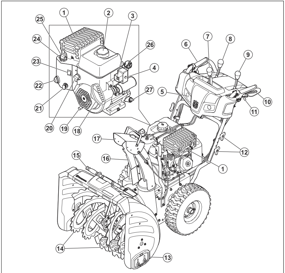
1. Lyddemper
