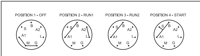
POSITIONS INTERRUPTEUR
