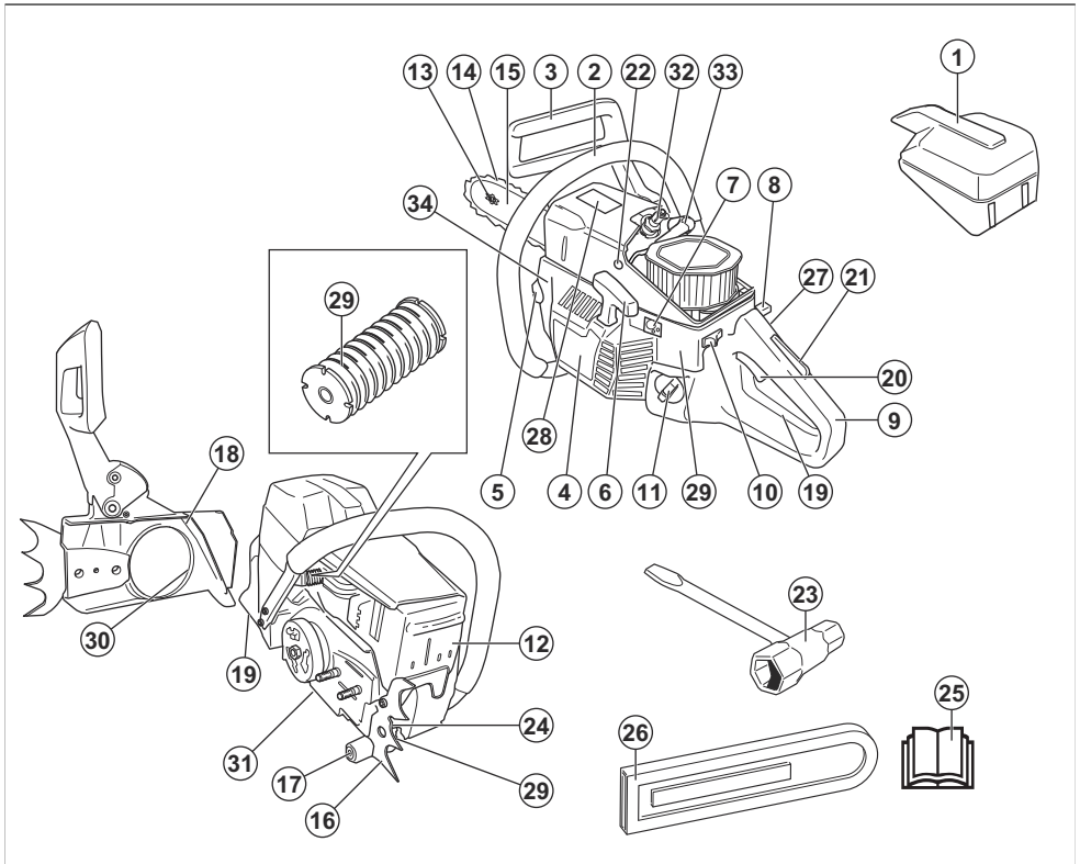
1. Couvercle de filtre à air
