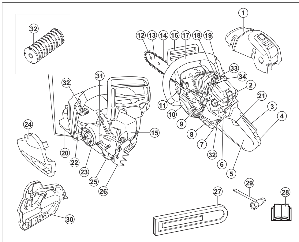
1. Cilinderkap
